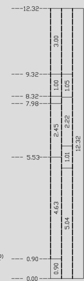
PROSPETTO NORD-EST
